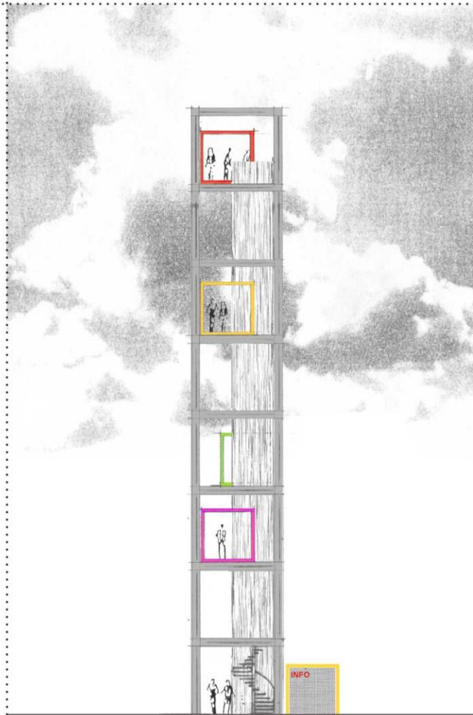
Ansicht NORDEN M 1:100
